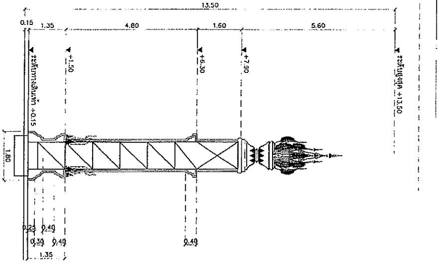
รูปตัดโค้งสร้างด้านข้าง มาตราส่วน 1 : 75
